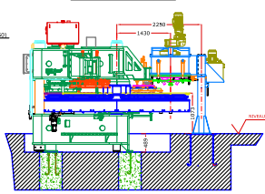
VUE EN ELEVATION DOSEUR (E1120)
