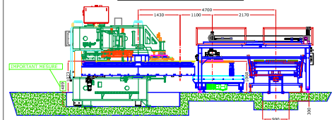
VUE EN ELEVATION PRESSE-PELLE EXTRACTRICE (E120)
