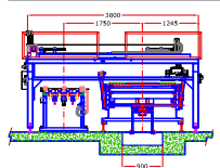
VUE EN ELEVATION EXTRACTEUR A VENTOUSES PRODUITS SECS (E120)
